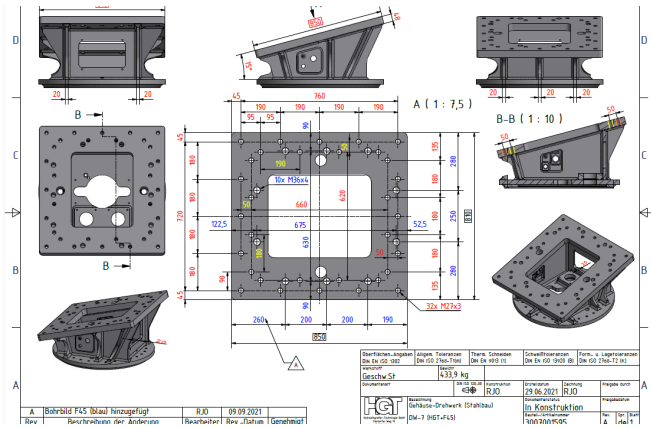
Ansicht 1
