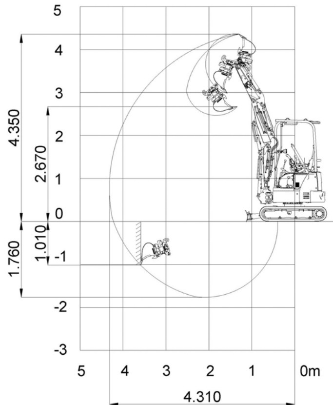
Bereichskurve gilt für QQR30 mit Tieföffel GB02P-030
