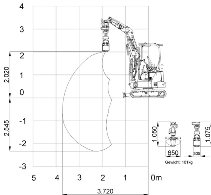
Bereichskurve gilt für QQR30 mit Tieföffel GB02P-030
