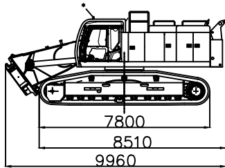
Grundmaschine ohne Ballast
