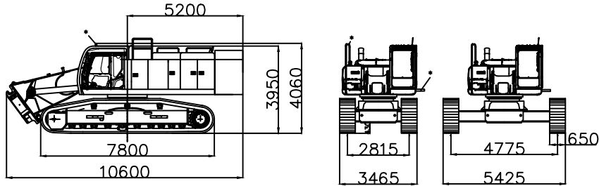
Grundmaschine mit Ballast
