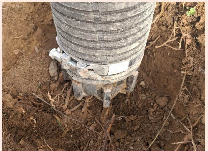
Oszillierender Saugstutzen löst das Material schonend
